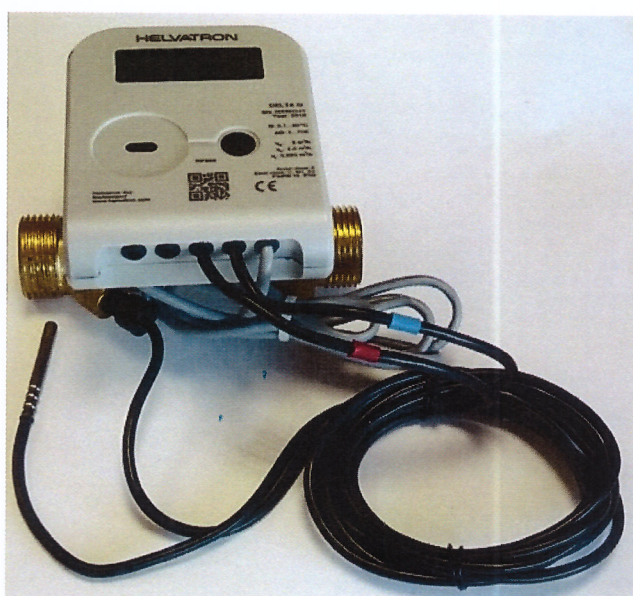
Fig.1.Heat meter DELTA III
