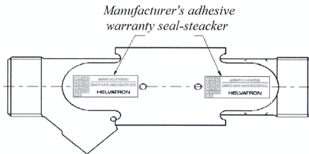
Fig. 7. Sealing of flow sensor q_p = 0,6/1,0/1,5/2,5 \text{ m}^3/\text{h}
