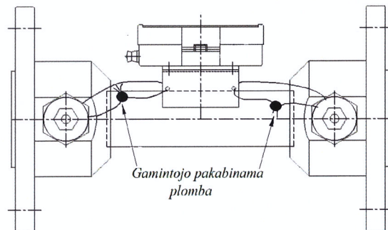
7 pav. Srauto jutiklio matavimo ruožo q_p = 3,5/6 \text{ m}^3/\text{h} plombavimas
