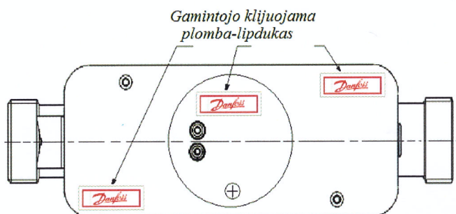
7 pav. Srauto jutiklio matavimo ruožo q_p = 3,5/6 \text{ m}^3/\text{h} plombavimas
