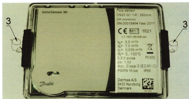
5 pav. Srauto jutiklio elektronikos bloko plombavimas
