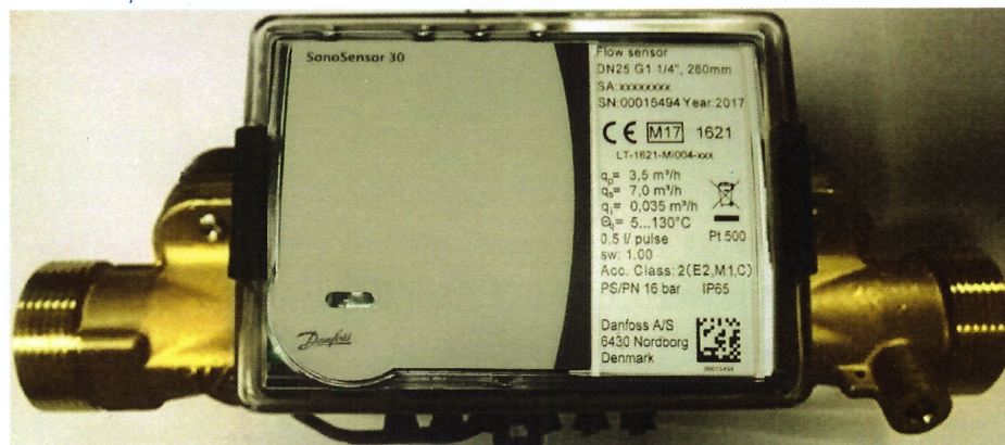
1 pav. Srauto jutiklis SonoSensor 30 (matavimo ruožas ir elektronikos blokas)
