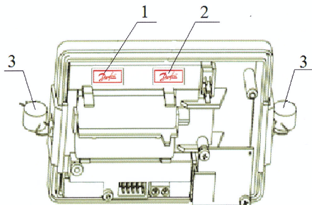
5 pav. Srauto jutiklio elektronikos bloko plombavimas
