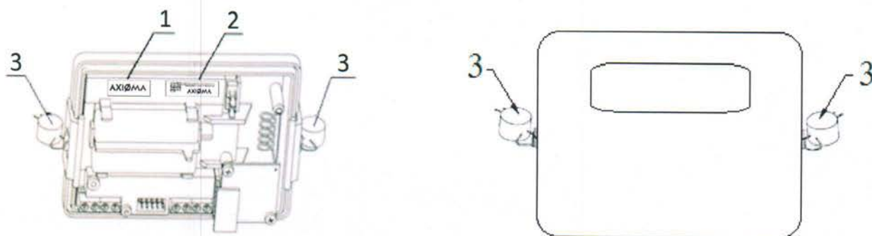
6 pav. Vandens skaitiklio QALCASONIC F1 skaičiuotuvo plombavimo schemas
