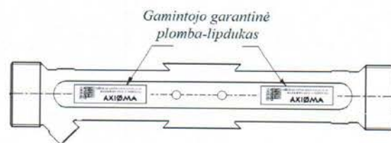
d) Vandens skaitiklio srauto jutiklio su prijungimu G1 \frac{1}{4} , G1 \frac{1}{2} , DN25, DN32 plombavimas (IP65 ir IP68, apvalaus skerspjūvio matavimo kanalas)
