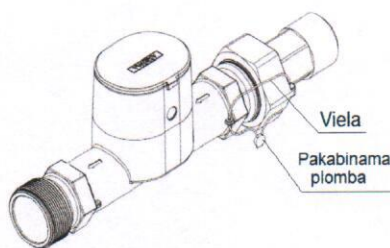
b) Skaitiklis su srieginiu prijungimu G 1\frac{1}{4} , G 1\frac{1}{2} , G 2
