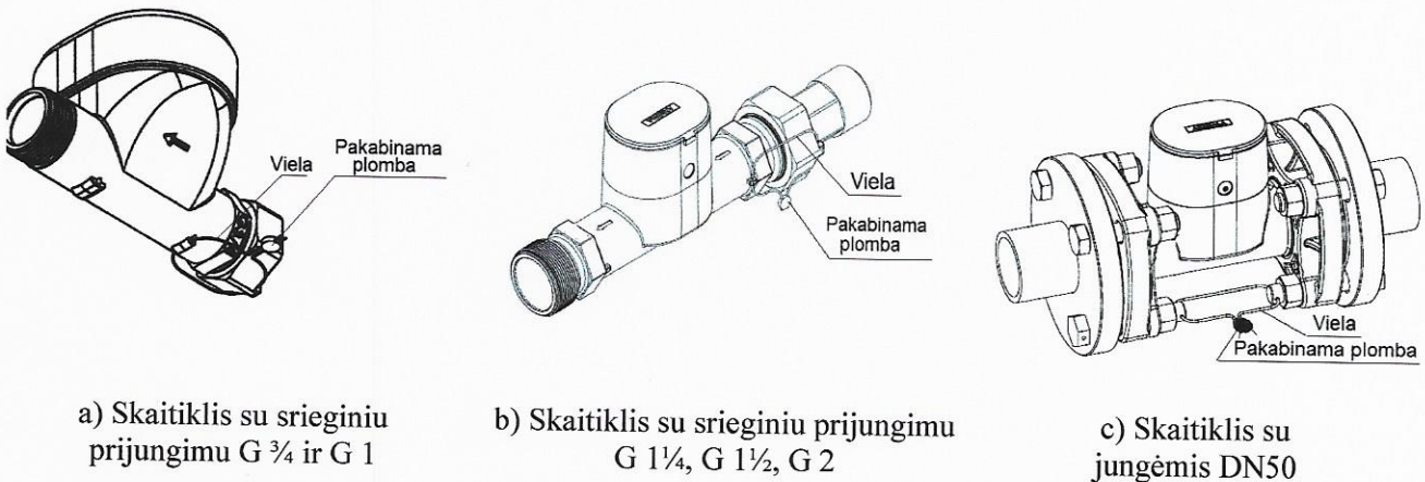
6 pav. Vandens skaitiklio QALCASONIC W1 plombavimas po įrengimo
