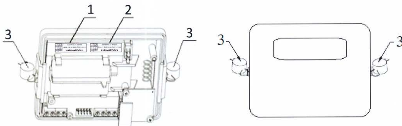
4 pav. Vandens skaitiklio H_2O skaičiuotuvo plombavimo schemos
