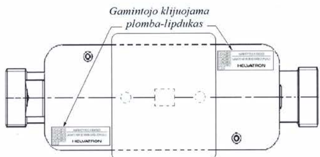
b) Vandens skaitiklio srauto jutiklio su prijungimu G 1\frac{1}{4} , DN25 plombavimas
