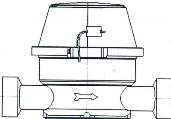
2 pav. Vandens skaitiklio JETO plombavimas
