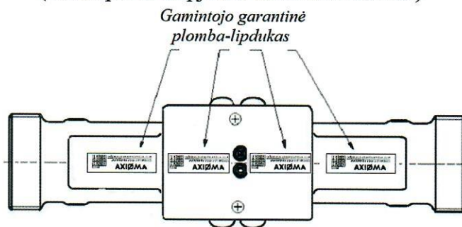
b) srauto jutiklio q_p = 3,5/6 \text{ m}^3/\text{h} plombavimas (trikampio skerspjūvio matavimo kanalas)
