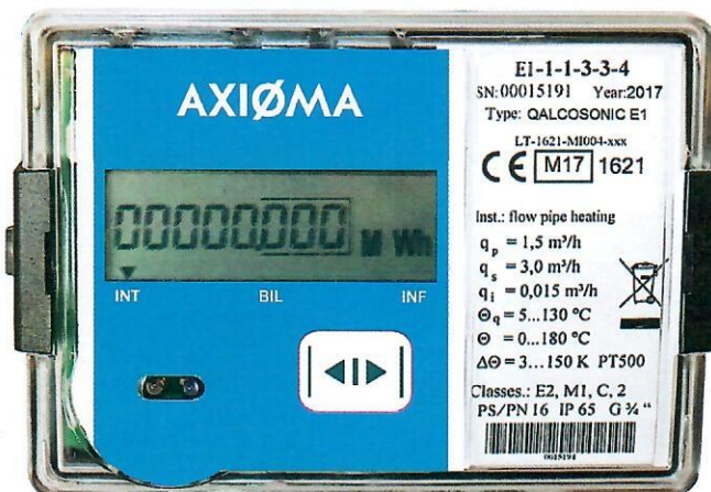
2 pav. Šilumos skaitiklio QALCOSONIC E1 skaičiuotuvas
