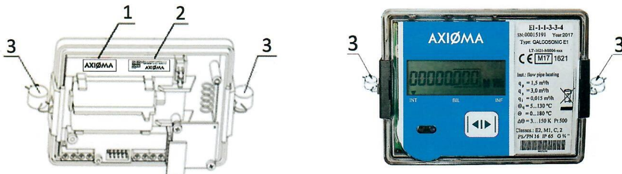
4 pav. Šilumos skaitiklio skaičiuotuvo plombavimas
