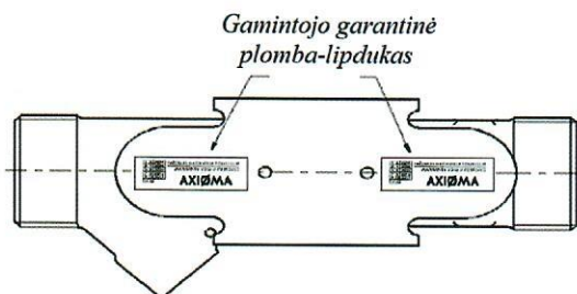
a) srauto jutiklio q_p = 0,6/1,0/1,5/2,5 \text{ m}^3/\text{h} plombavimas
