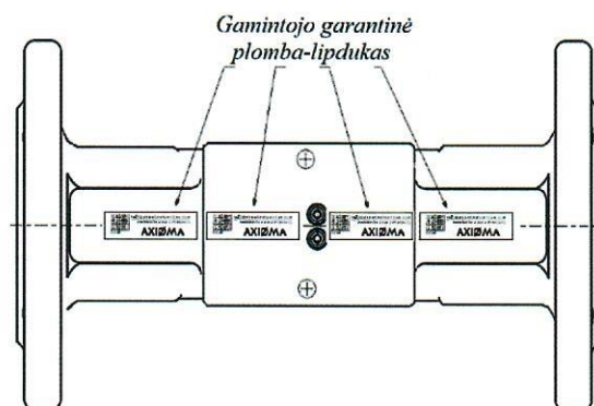
e) srauto jutiklio q_p = 15/25/40/60 \text{ m}^3/\text{h} plombavimas
