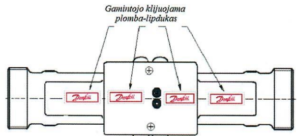
d) Srauto jutiklio q_p = 10,0 \text{ m}^3/\text{h} plombavimas
