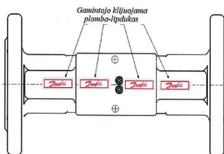
e) Srauto jutiklio q_p = 15/25/40/60 \text{ m}^3/\text{h} plombavimas
