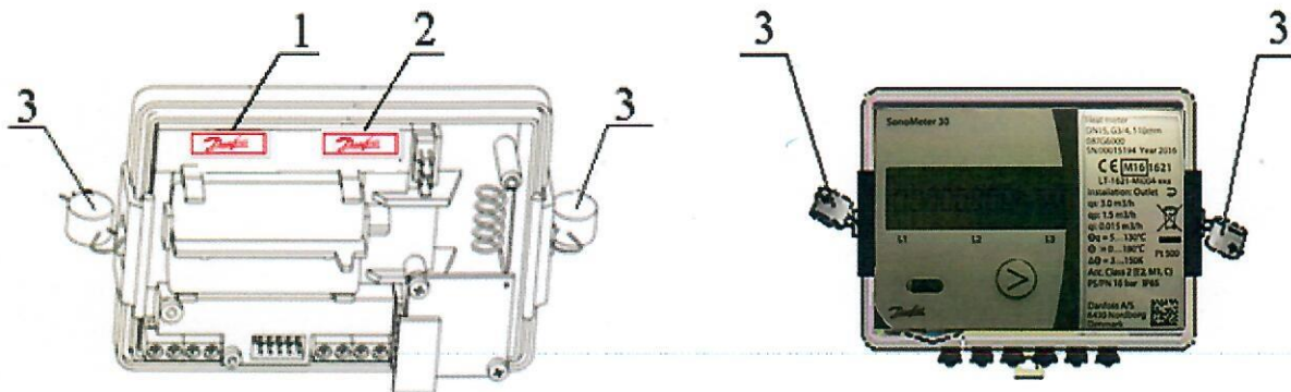
4 pav. Šilumos skaitiklio skaičiuotuvo plombavimas
