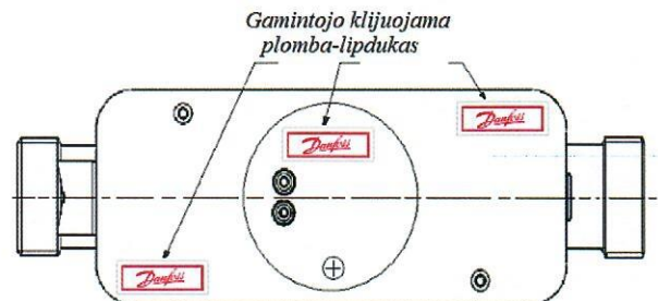
b) Srauto jutiklio q_p = 3,5/6,0 \text{ m}^3/\text{h} plombavimas (trikampio skerspjūvio matavimo kanalas)
