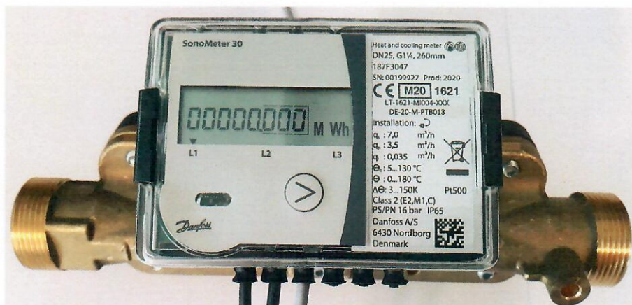
1 pav. Šilumos skaitiklis SonoMeter 30 (skaičiuotuvas ir srauto jutiklis)
