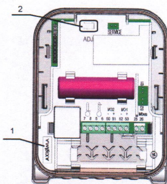
7 pav. Sudėtinio prietaiso skaičiuotuvo papildomas plombavimas
