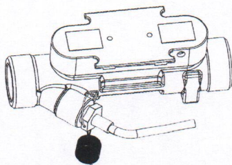
a) Temperatūros zondo, montuojamo srauto jutiklio korpusė plombavimas
