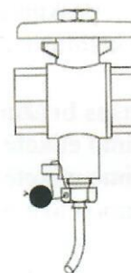
c) Temperatūros zondo, montuojamo rutulinėje sklendėje plombavimas
