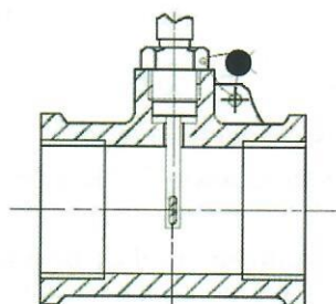
b) Temperatūros zondo, montuojamo trišakyje plombavimas
