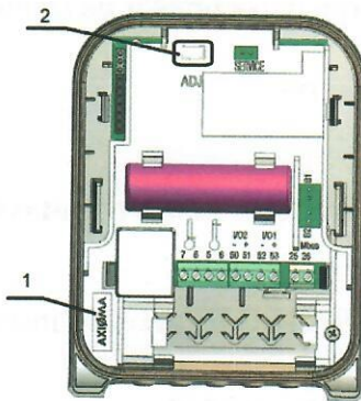
7 pav. Sudėtinio prietaiso skaičiuotuvo papildomas plombavimas
