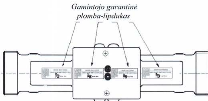
9 pav. Srauto jutiklio q_p = 10/15/25/40/60 \text{ m}^3/\text{h} plombavimas
