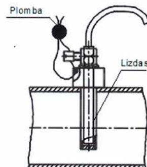
11 pav. PL tipo temperatūros zondu plombavimas
