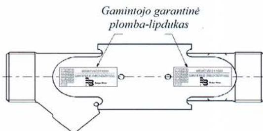
7 pav. Srauto jutiklio q_p = 0,6/1,0/1,5/2,5 \text{ m}^3/\text{h} plombavimas
