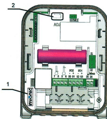
7 pav. Skaitiklio INVONIC 2M skaičiuotuvo papildomas plombavimas
