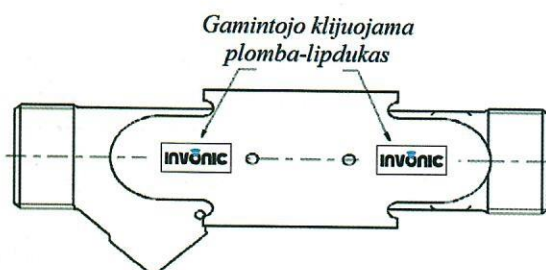
a) srauto jutiklio q_p = 0,6/1,0/1,5/2,5 \text{ m}^3/\text{h} plombavimas
