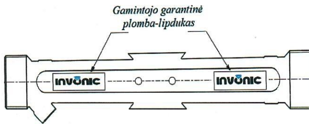
c) srauto jutiklio q_p = 3,5 \text{ m}^3/\text{h} plombavimas (apvalaus skerspjuvio matavimo kanalas)
