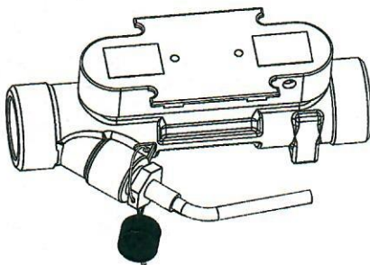
a) Temperatūros zondo, montuojamo srauto jutiklio korpuse plombavimas
