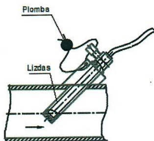
10 pav. PL tipo temperatūros zondu plombavimas
