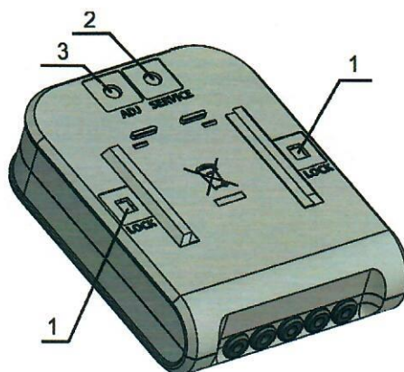
6 pav. Šilumos energijos skaitiklio INVONIC 2 (2M) skaičiuotuvo plombavimas
