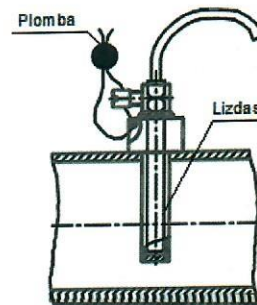
10 pav. PL tipo temperatūros zondu plombavimas
