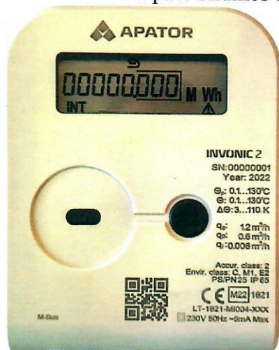
a) Šilumos energijos skaitiklio INVONIC 2 skaičiuotuvas b) Šilumos energijos skaitiklio INVONIC 2M skaičiuotuvas 2 pav. Šilumos energijos skaitiklio INVONIC 2 (2M) skaičiuotuvas
