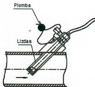
9 pav. PL tipo temperatūros zondu plombavimas
