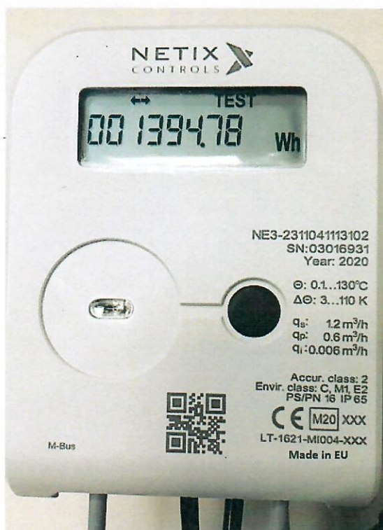
1 pav. Šilumos energijos skaitiklio NE3 skaičiuotuvas
