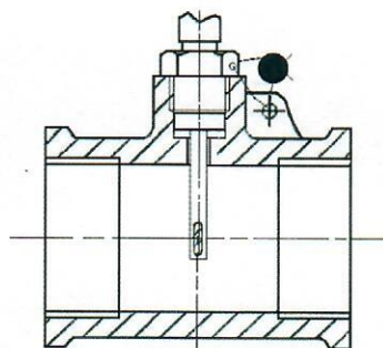
9 pav. PL tipo temperatūros zondu plombavimas
