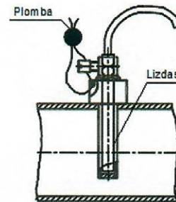
9 pav. PL tipo temperatūros zondu plombavimas
