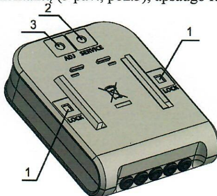
5 pav. Šilumos energijos skaitiklio skaičiuotuvo plombavimas
