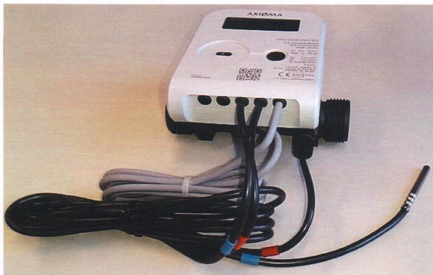
1 pav. Šilumos energijos skaitiklis QALCASONIC E4
