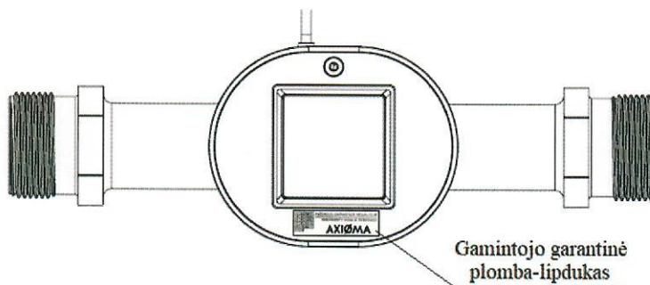
6 pav. Srauto jutiklio q_p = 3,5/6/10/15 \text{ m}^3/\text{h} plombavimas
