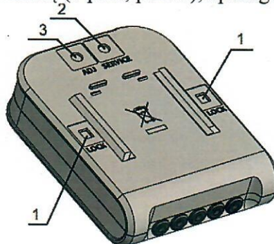
4 pav. Šilumos energijos skaitiklio skaičiuotuvo plombavimas
