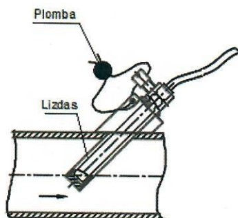
7 pav. PL tipo temperatūros zondu plombavimas
