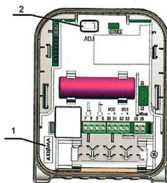
5 pav. Sudėtinio prietaiso skaičiuotuvo papildomas plombavimas
