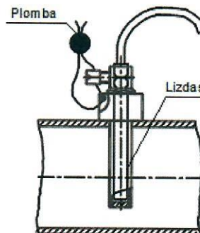
7 pav. PL tipo temperatūros zondu plombavimas
