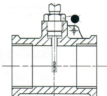
b) Temperatūros zondo, montuojamo trišakyje plombavimas
