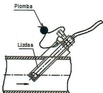
7 pav. PL tipo temperatūros zondu plombavimas
