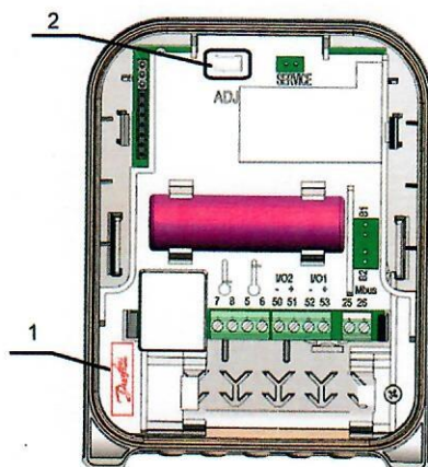
6 pav. Sudėtinio prietaiso skaičiuotuvo papildomas plombavimas
