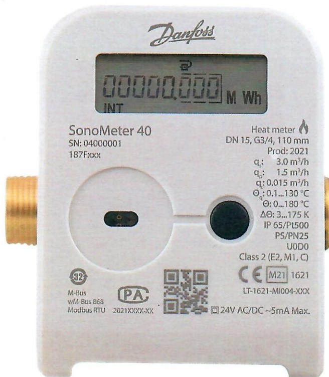
1 pav. Šilumos energijos skaitiklis SonoMeter 40
