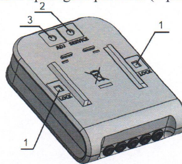
5 pav. Skaitiklio skaitliuotuvo plombavimas
