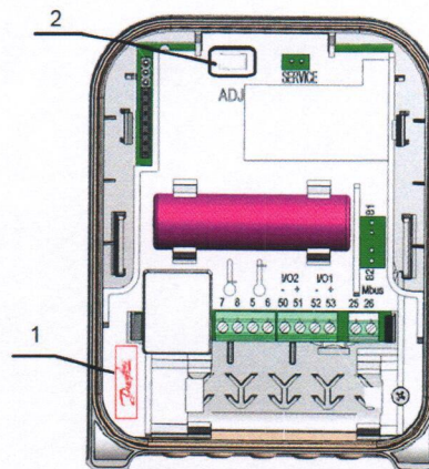
6 pav. Sudėtinio prietaiso skaitliuotuvo papildomas plombavimas
