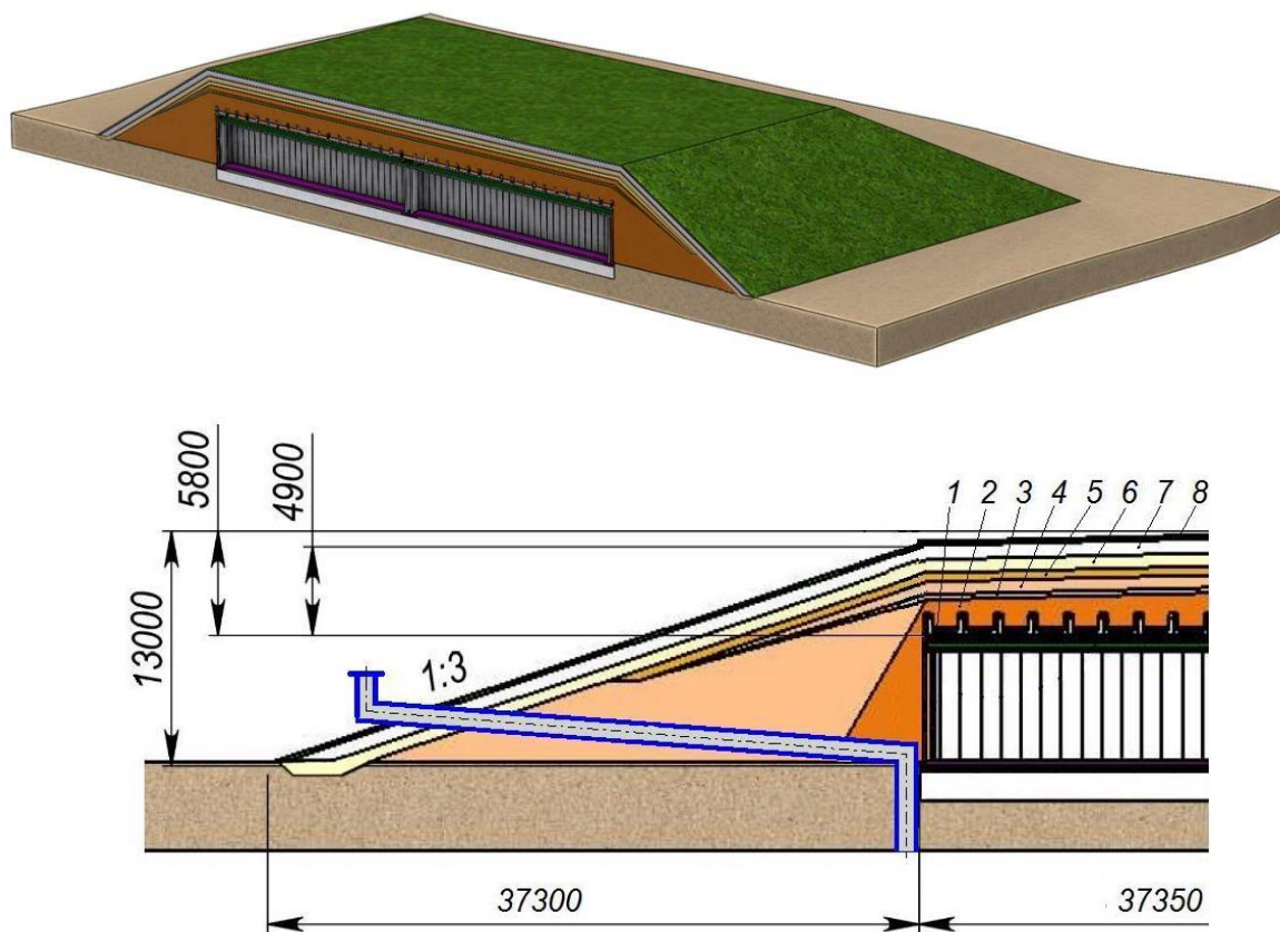
S2 pav. Saugyklos, pertvarkytos į atliekyną, vaizdas ir 5,8 m storio inžinerinio barjero sandara (pjūviai): 1 – dujų pašalinimo sluoksnis (0,2 m smėlio); 2 – izoliacinis molio sluoksnis (1,5-2,4 m); 3 – drenazo sluoksnis (0,3 m žvyringo smėlio); 4 – apsauginis molio sluoksnis (0,7 m); 5–7 – drenazo sluoksniai (0,6 m smėlio, 0,6 m žvyro ir 0,8 m skaldos); 8 – 0,2 m storio augalinis sluoksnis
