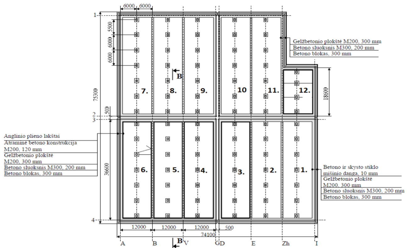
1.4 pav. 158 pastato kanjonų išdėstymo planas
