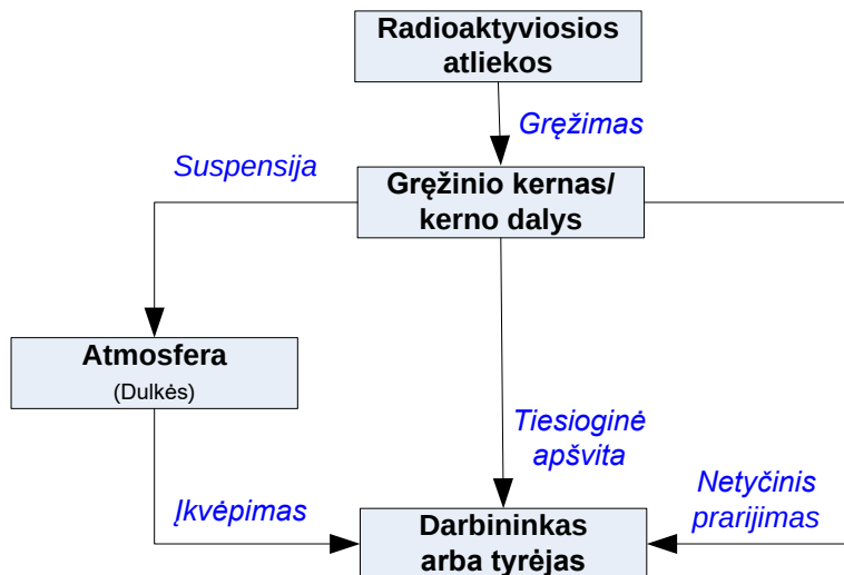
4.29 pav. Konceptualus radionuklidų sklaidos ir apšvitos trasų, į gręžimo scenarijaus atveju, modelis
