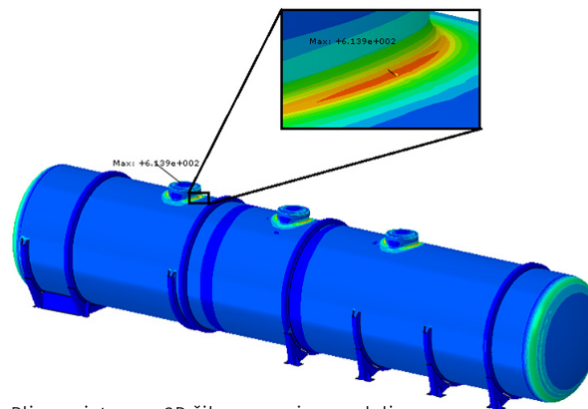
Plieno cisternos 3D šilumos mainų modelis
