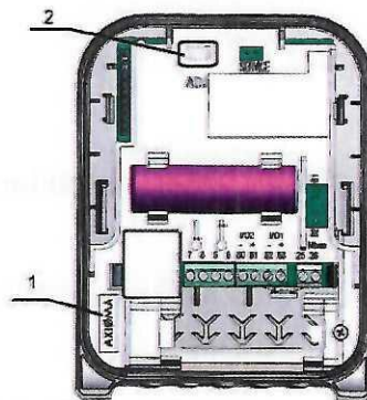
7 pav. Sudėtinio prietaiso skaičiuotuvo papildomas plombavimas
