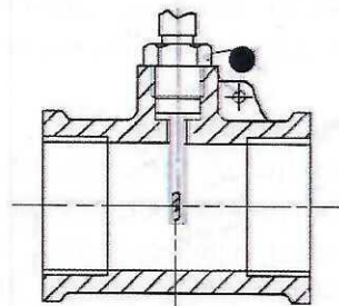
b) Temperatūros zondo, montuojamo trišakyje plombavimas
