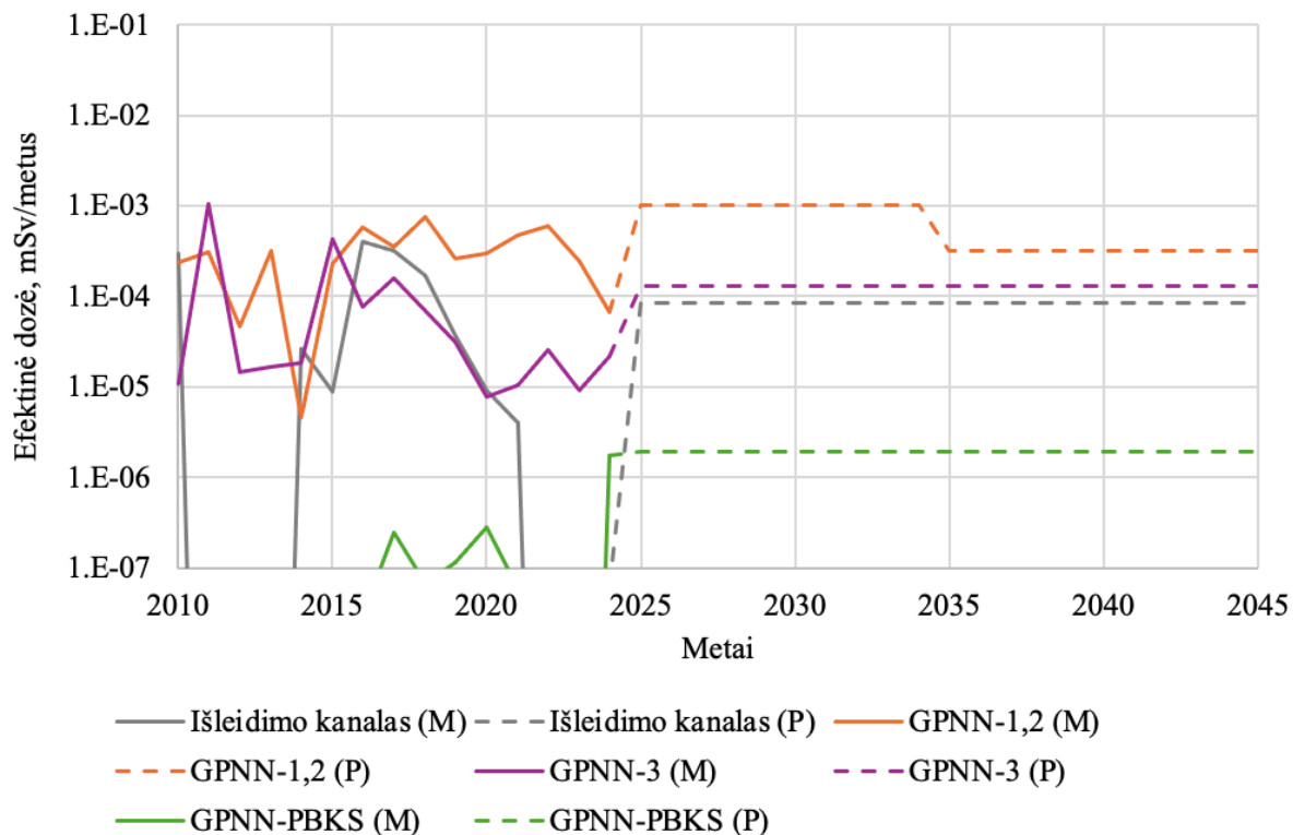
4.9-5 pav. Radioaktyviųjų išmetimų į aplinkos vandenį per atskirus nuotekų išleidimo kanalus lemta gyventojų metinė efektinė dozė. (M) – monitoringo duomenys, (P) prognozuojami išmetimai
