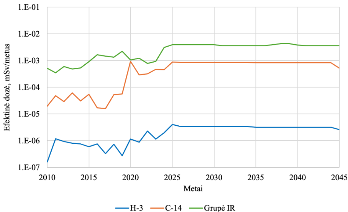
4.9-7 pav. H-3, C-14 ir IR grupių radionuklidų išmetimo į aplinkos orą lemta gyventojų metinė efektinė dozė
