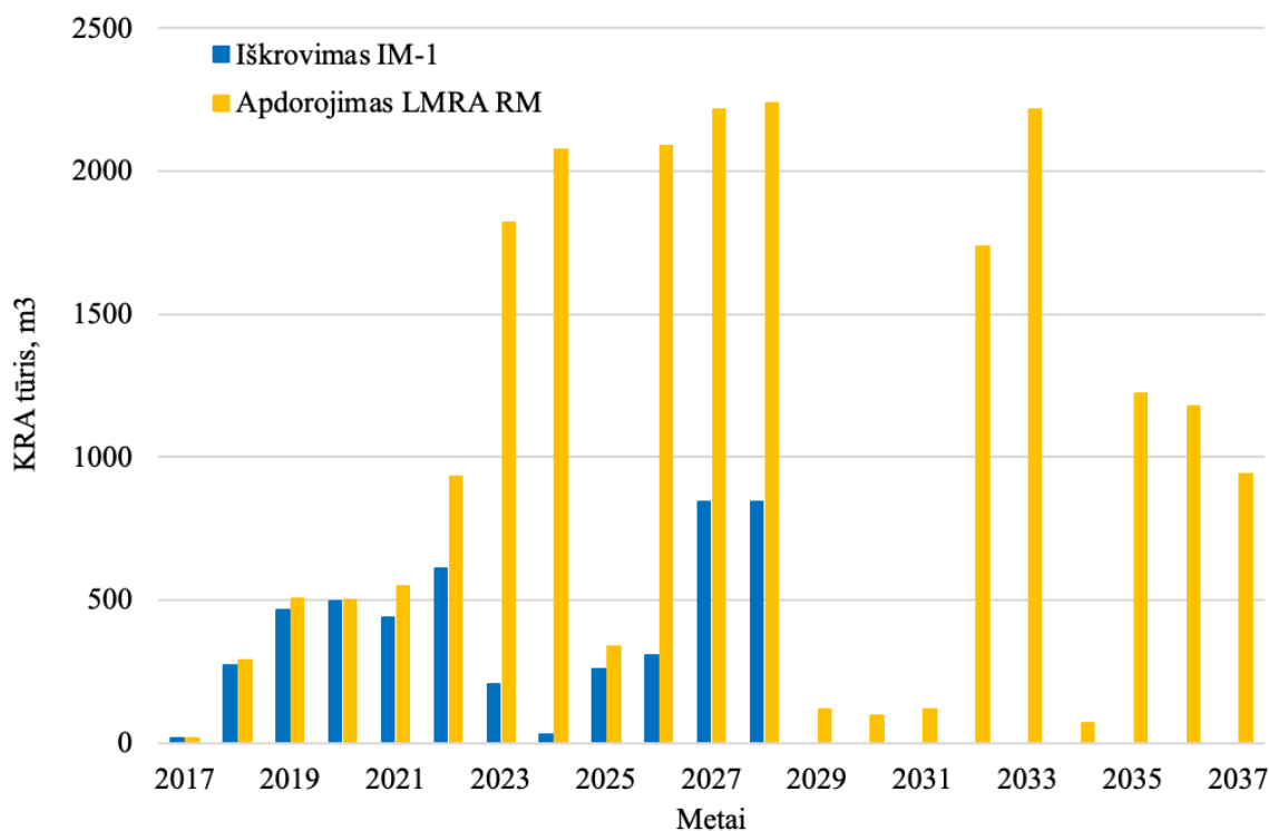
3.2-4 pav. G1 grupės KRA išėmimas su IM-1 iš pastatų Nr. 155/1 ir Nr. 155 bei KRA pradinis apdorojimas LMRA rūšiavimo modulyje
