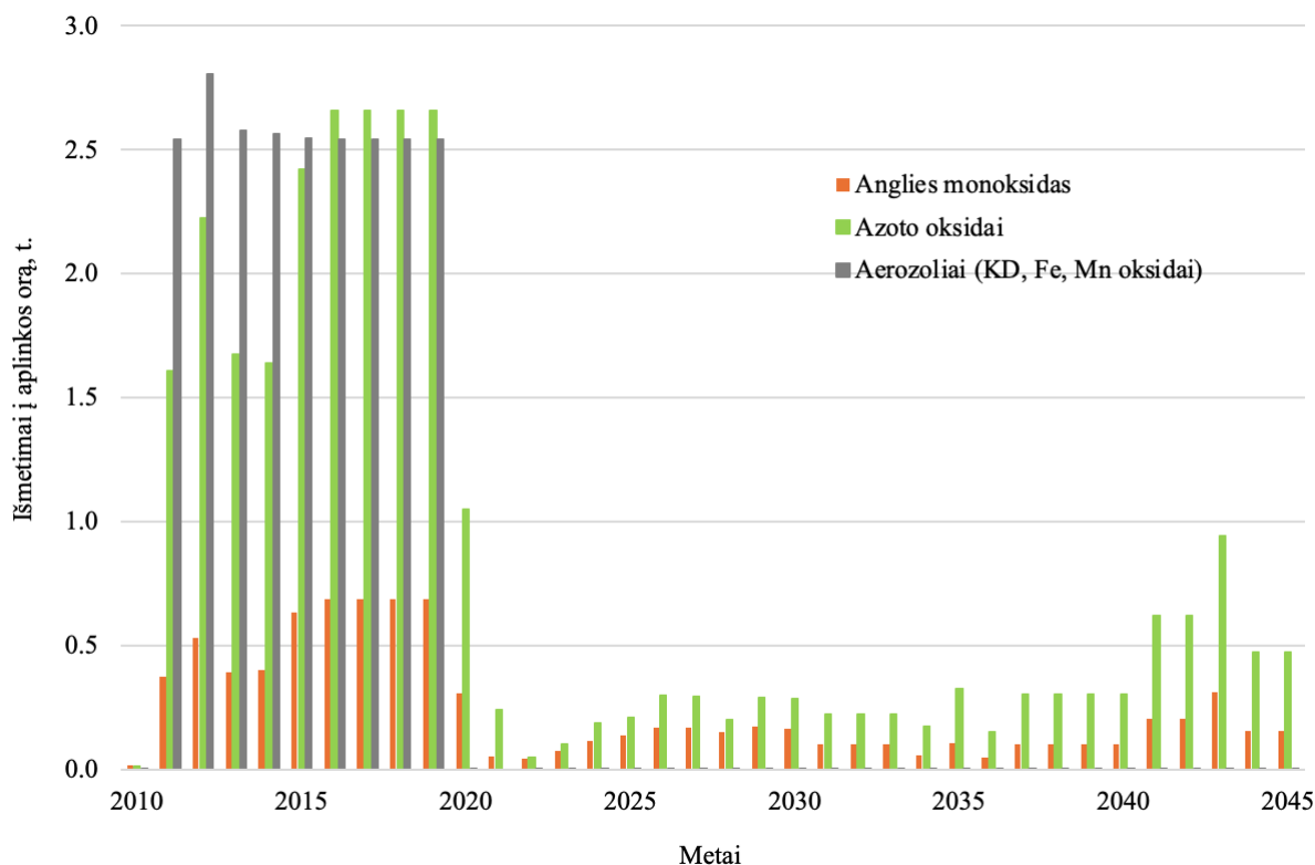
4.2-17 pav. IirPA projektuose įvertinti atskirų teršalų išmetimai į aplinkos orą ir tolimesnėms IirPA veikloms prognozuojami atskirų teršalų išmetimai į aplinkos orą
