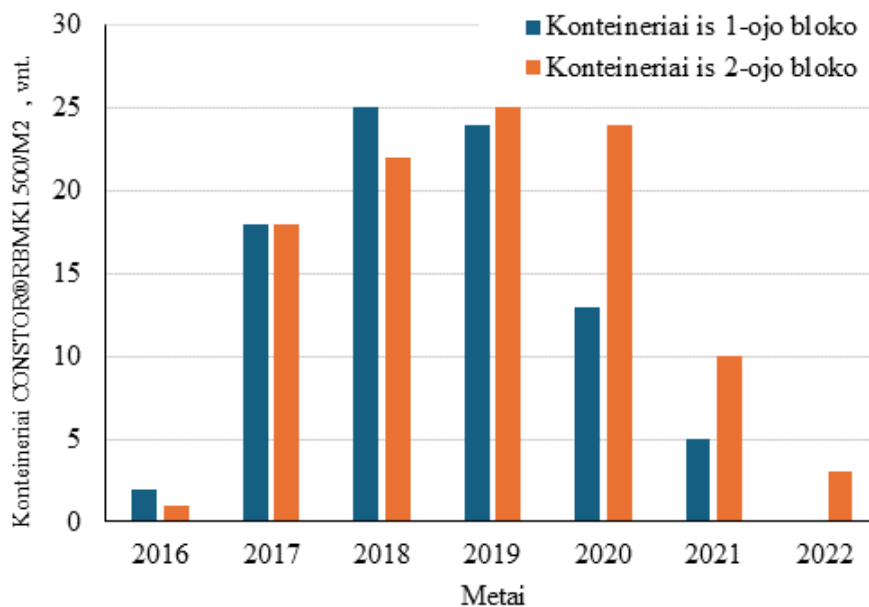
3.2-2 pav. Konteinerių CONSTOR®RBMK1500/M2 su PBK išvežimo ir patalpavimo LPBKS-2 eiga
