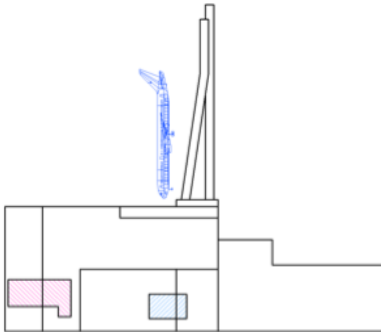
5.2-1 pav. 2-ojo energijos bloko reaktorius pastatas, vaizdas iš rytinės pusės. Pastato ir lėktuvo schemas pavaizduotos tuo pačiu masteliu
