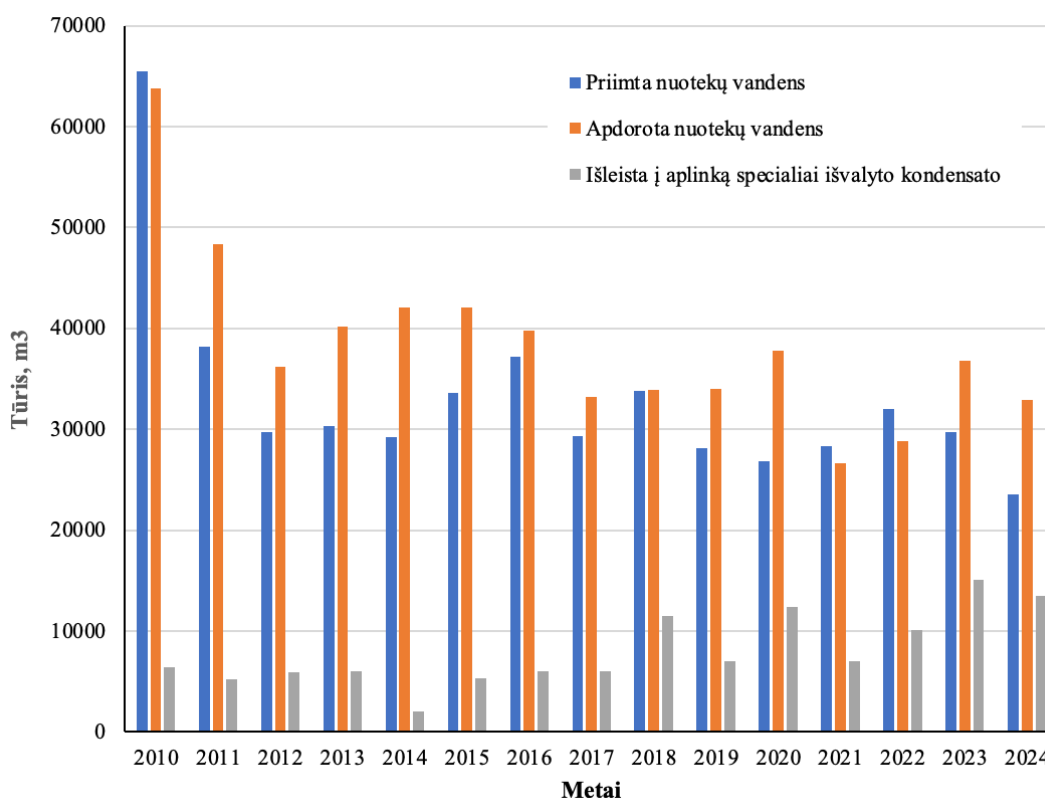
3.1-4 pav. IAE SKRA apdoravimo komplekse surinktų ir apdorotų nuotekų vandens tūriai bei į aplinką išleisto specialiai išvalyto kondensato tūriai
