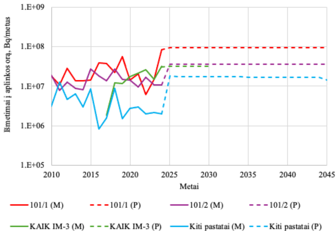
4.2-19 pav. IR grupės radionuklidų išmetimas iš atskirų IAE pastatų, (M) – monitoringo duomenys, (P) – prognozuojami išmetimai
