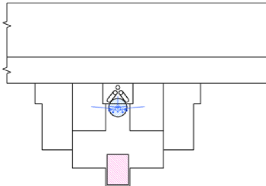
5.2-2 pav. 2-ojo energijos bloko reaktorius pastatas, vaizdas iš viršaus. Pastato ir lėktuvo schemas pavaizduotos tuo pačiu masteliu.
