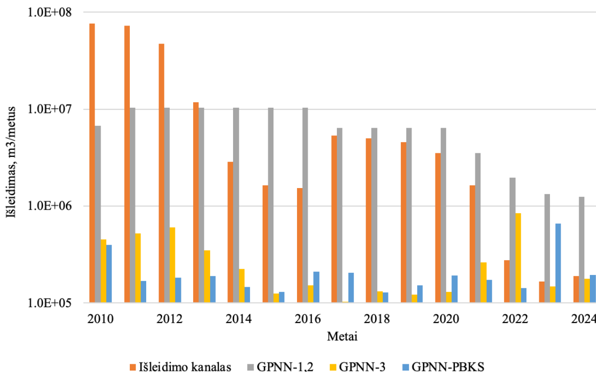
4.1-6 pav. Bendras technologinio ir perteklinio vandens išleidimas per atskirus kanalus į Drūkšių ežerą
