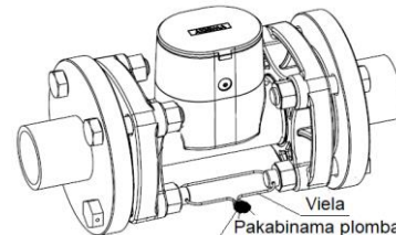
c) Skaitiklis su jungėmis DN50
