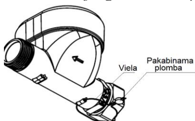
a) Skaitiklis su srieginiu prijungimu G 3/4 ir G 1
