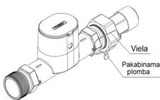
b) Skaitiklis su srieginiu prijungimu G 1 1/4, G 1 1/2, G 2
